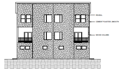
Elevation 4 - e
